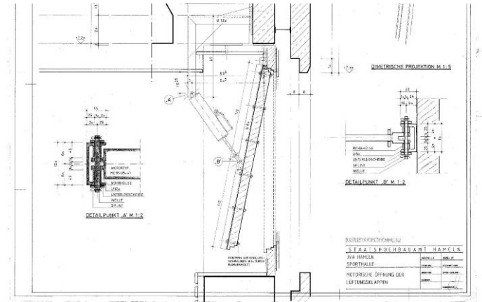
(8) Vorhandener Detailplan (Ordner „Elektro“)
