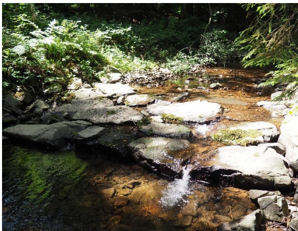
Abbildung 11: Objekt-Nr. 018 - Blocksteinrampe - Blickrichtung stromaufwärts
