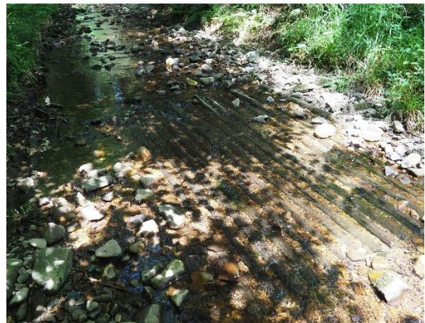
Abbildung 6: Objekt-Nr. 010 – Grundschwelle (Holz) - Blickrichtung stromabwärts
